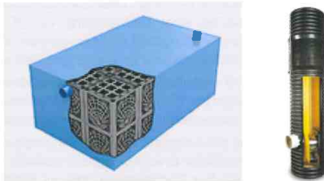
Abb. 13 Rigolenfüllkörper mit Kunststoffummantelung und Drosselschacht
